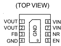
VDFN-8L 3x3
